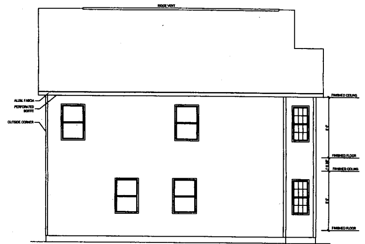
LEFT ELEVATION SCALE: 1/8"=1'-0"
