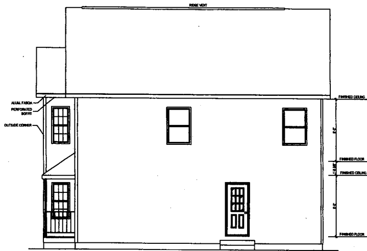
RIGHT ELEVATION SCALE: 1/8"=1'-0"
