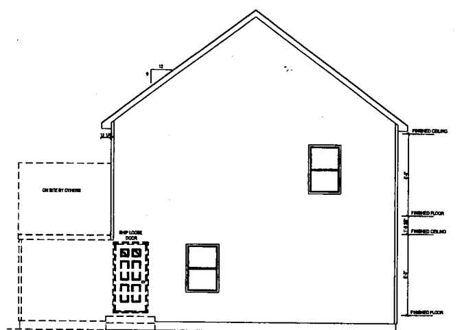
GABLE ELEVATION SCALE: 1/8"=1'-0"
