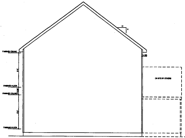
GABLE ELEVATION SCALE: 1/8"=1'-0"
