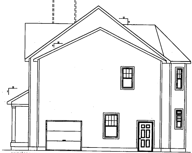
RIGHT SIDE ELEVATION SCALE: 1/8" = 1'-0"
