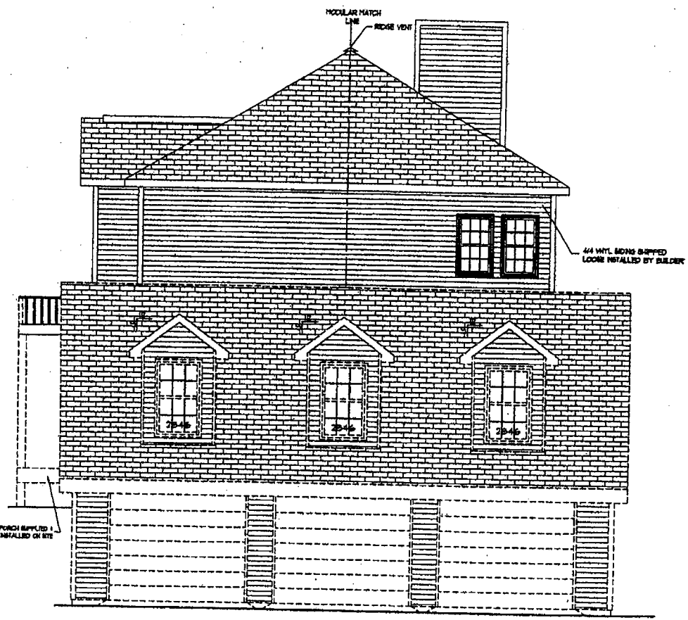
RIGHT ELEVATION
