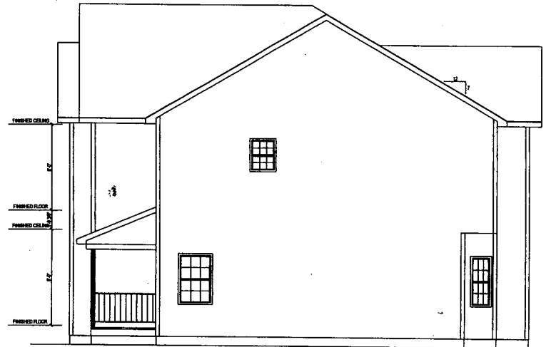
RIGHT ELEVATION SCALE: 1/8"=1'-0"
