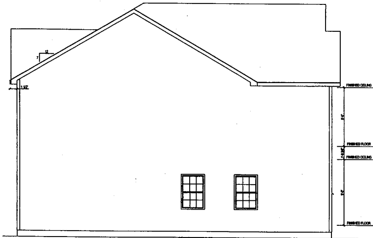
LEFT ELEVATION SCALE: 1/8"=1'-0"
