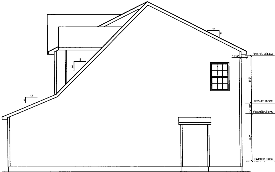
RIGHT ELEVATION
