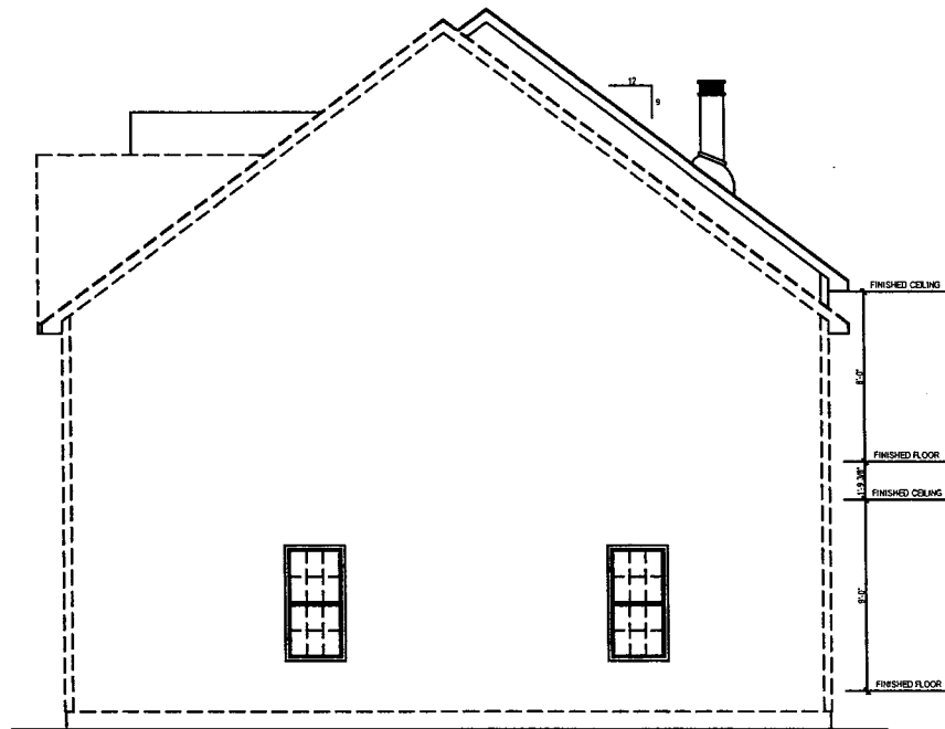
RIGHT ELEVATION
